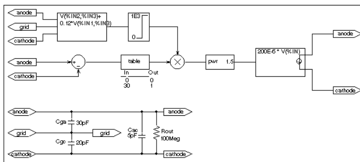
Figure 46 Triode circuit.
