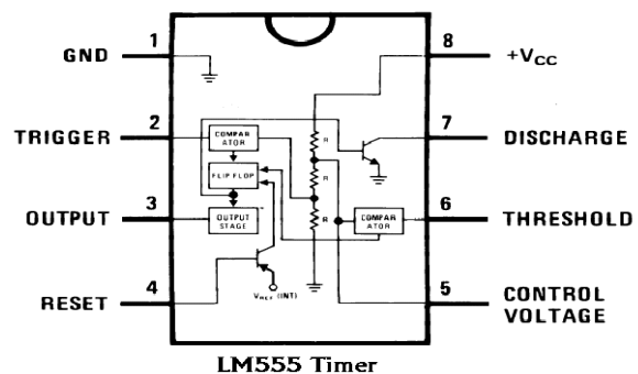
Fig. 11 LM 555 Timers
