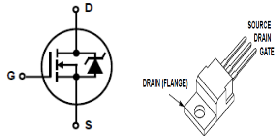
Fig. 10 Power MOSFET / IRF 540
