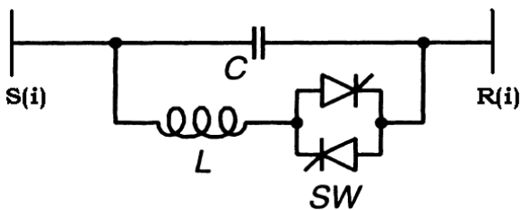
Fig.1 TCSC Module
