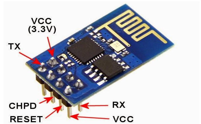
Fig3 -ESP8266 wifi module
